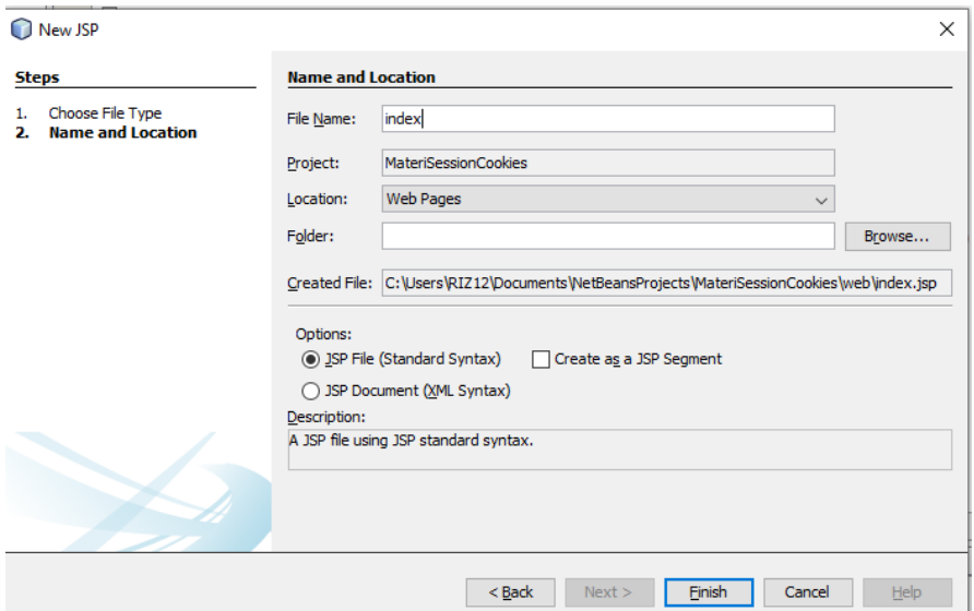
Gambar 199. Mengubah Nama
