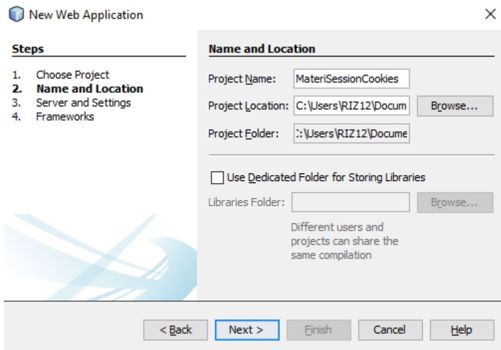
Gambar 196. Mengubah Nama
