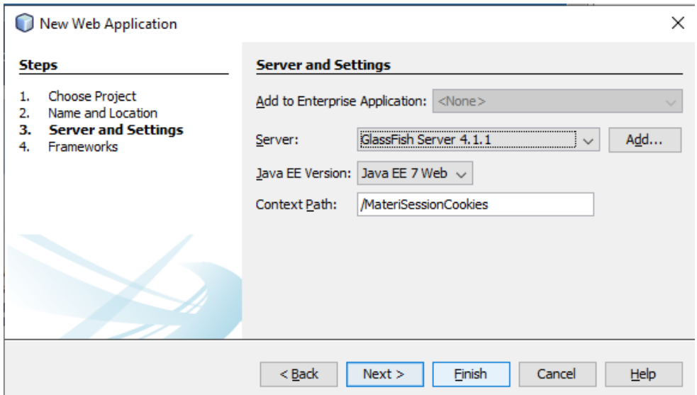
Gambar 197. Mengatur Server
