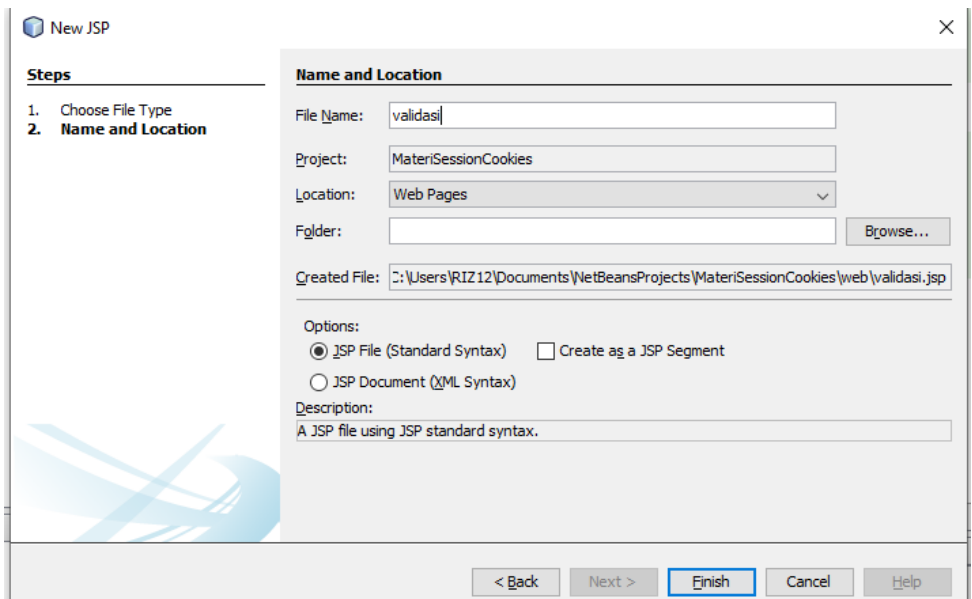
Gambar 203. Mengubah Nama
